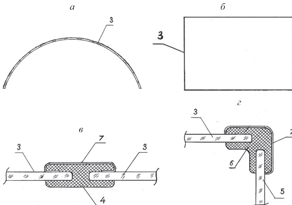
Рисунок 3 - Крепление стеклянных элементов ПО: а - прозрачного стеклянного ограждения; б - корытабассейна; в - крепление в ряду; г - крепление вид в торце.
