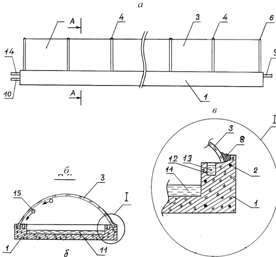
Рисунок 2 - Конструкция малометаллоемкого СОУ: а - схема конструктивного варианта разработанной СОУ; б, в - сечение корпуса СОУ.
