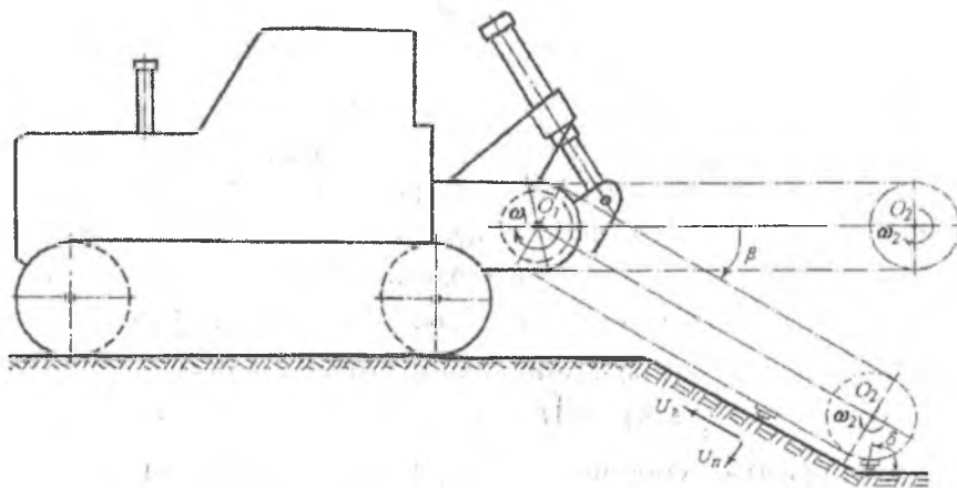
Рис.1. Внедрение ЦРО в массив природного камня
