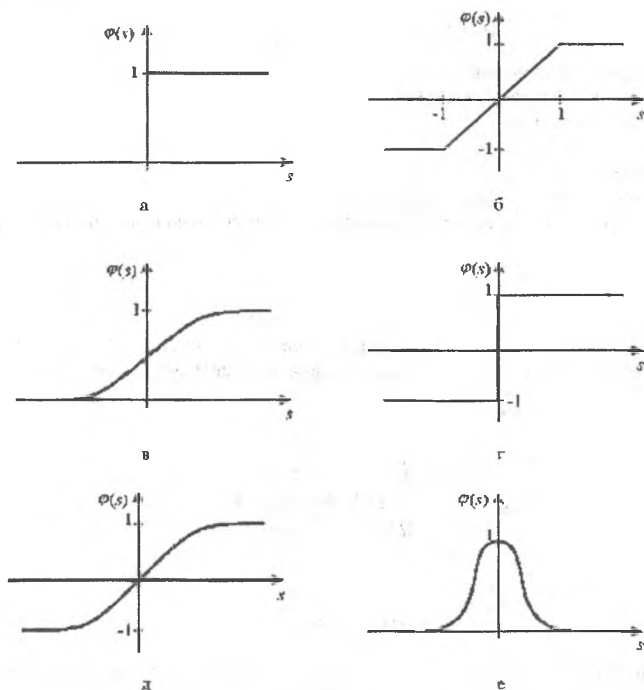
Рис. 3. Типы активационных функций.
