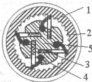
Рис. 1. Поворотный механизм с четырьмя собачками: 1-храповое кольцо; 2-плунжер; 3-пружина; 4-собачка; 5-храповой стержень.
