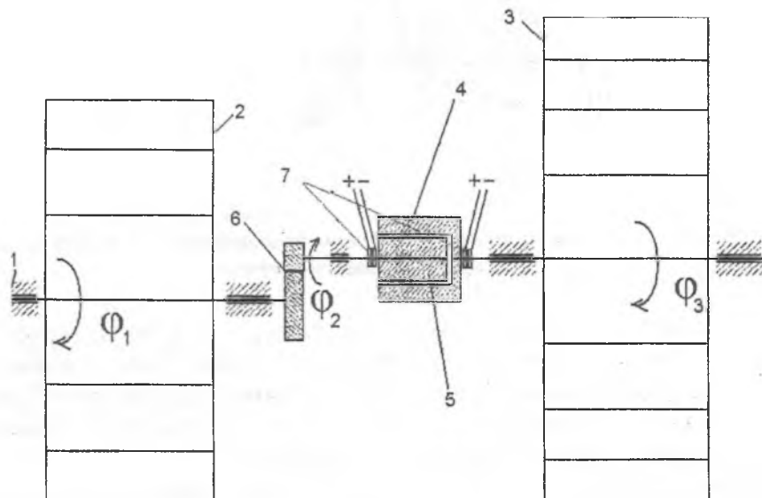
Рис. 1. Микро гидроэлектростанция на основе преобразователя энергии с двумя вращающимися частями.
