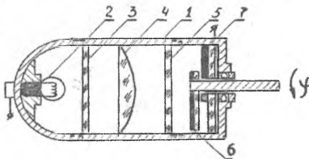
1-полый световод, 2-источник излучения, 3-фильтр, 4-диафрагма, 5-тепловой фильтр, 6-приемник излучения, 7-неподвижный приемник излучения
