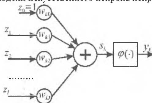
Рис. 2. Модель нейрона
