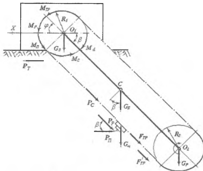
Рис.2. Динамическая модель ЦРО машины «Виктория» в процессе резания природного камня
